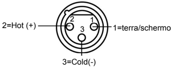
Connettore maschio XLR a 3 poli (visto dal lato della saldatura)
