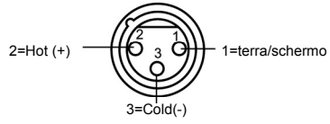
Connettore XLR a 3 poli (visto dal lato della saldatura)
